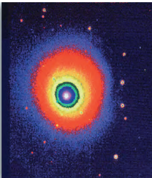
Nova
