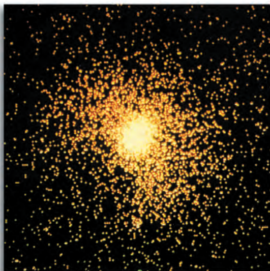
Pulsars
