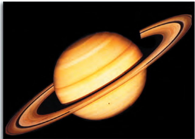
Saturn (NASA)
