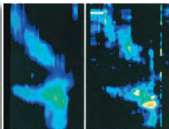
Pulsars
