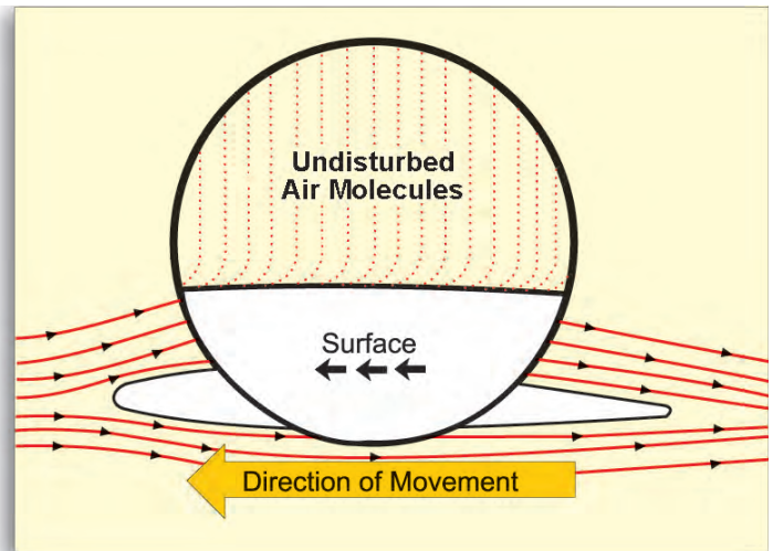
Viscous Drag
